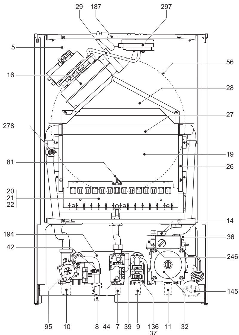
fig. 33 - Vista generale
