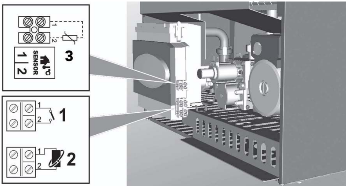
fig. 21 - Accesso alla morsettiera
