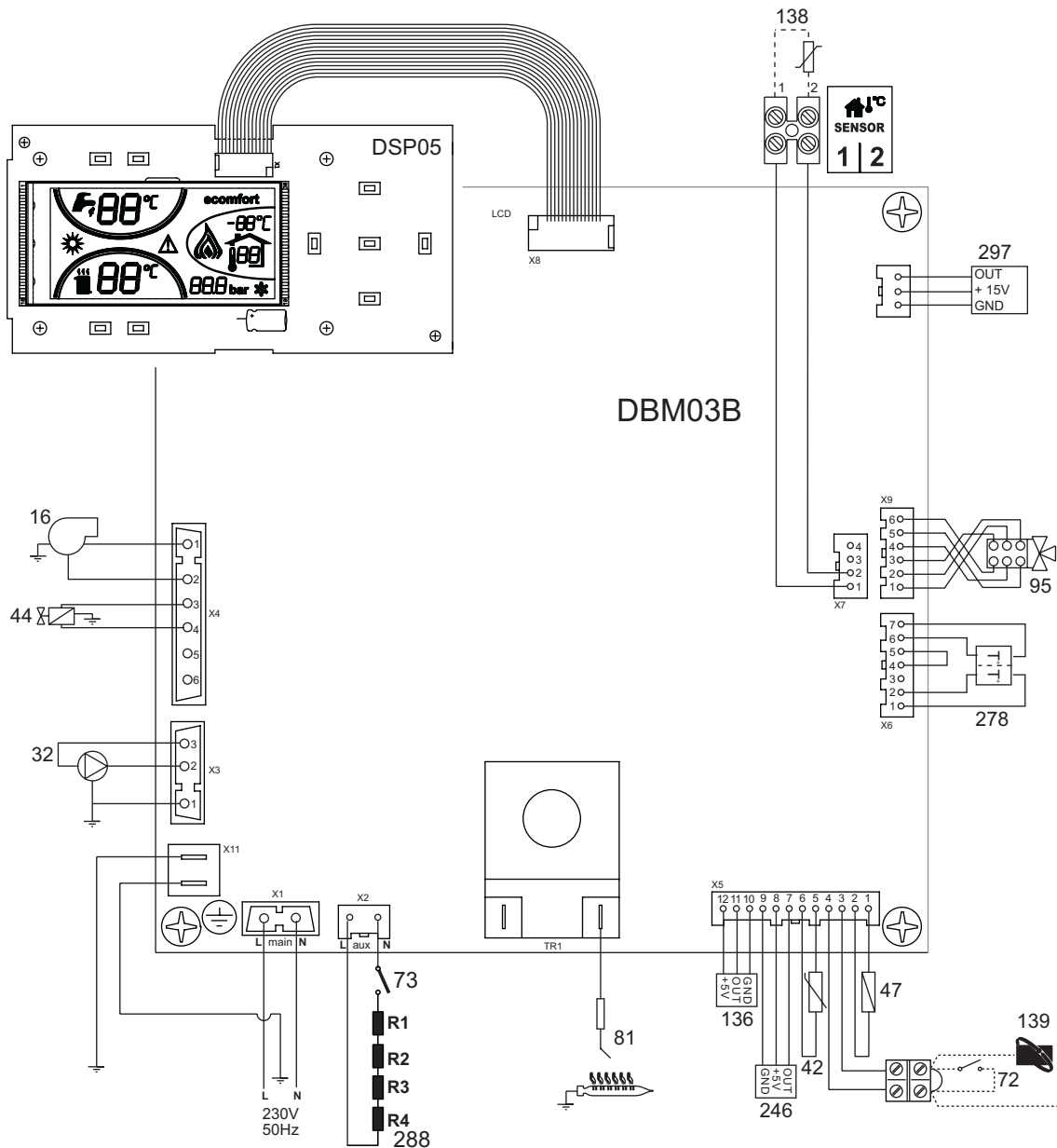
fig. 35 - Schema elettrico
