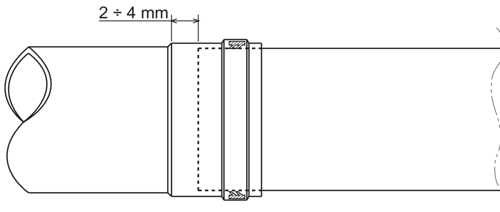
fig. 22 - Dilatazione
