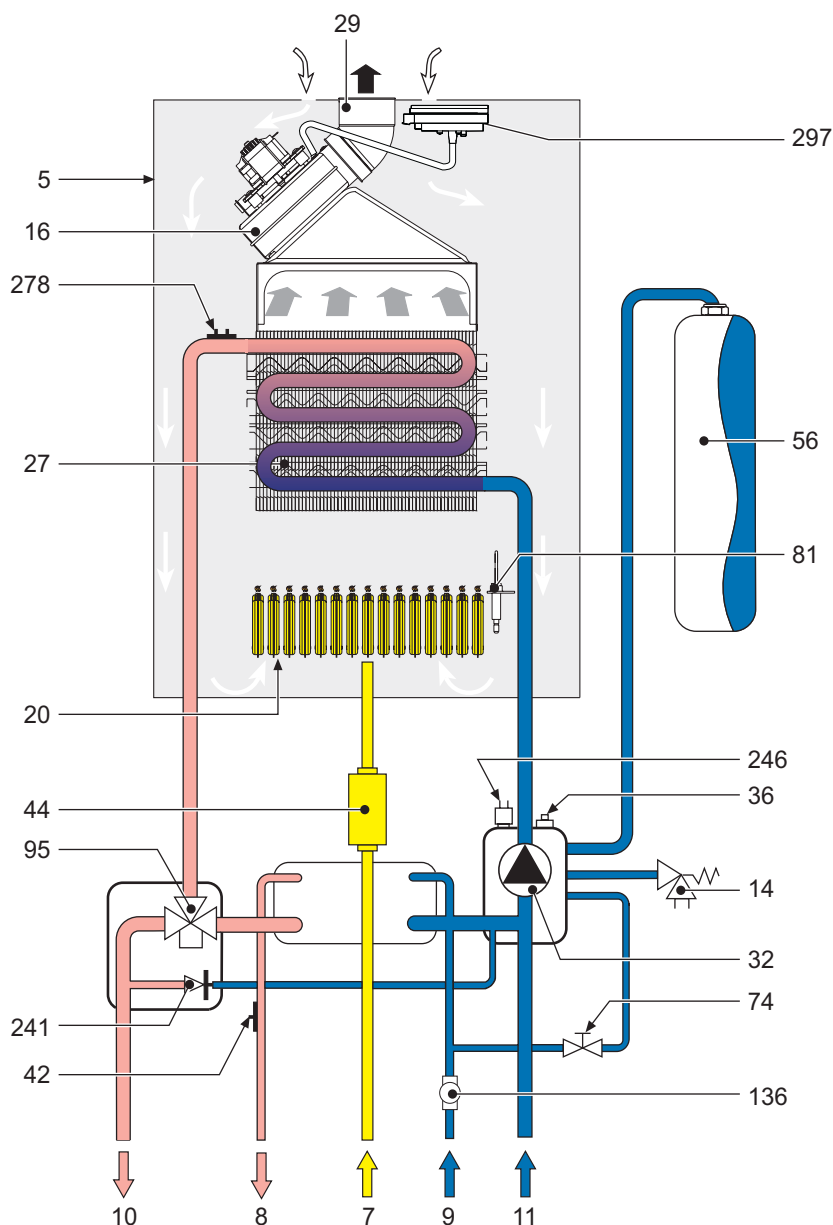
fig. 34 - Circuito idraulico
